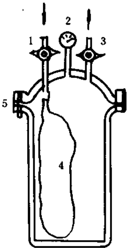
图 1 负压采气器采样图
