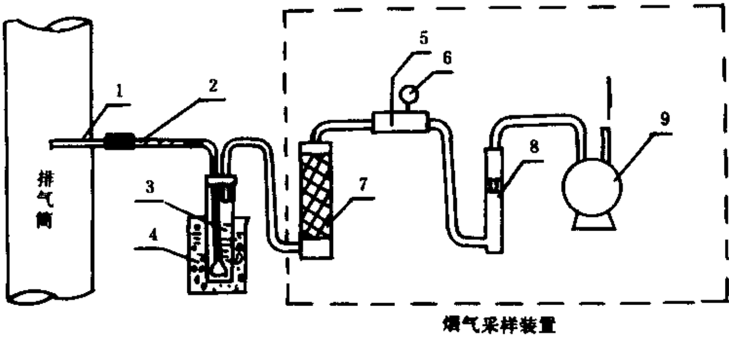
图 2 排气筒采样图
